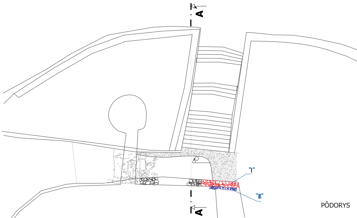
obr.01 zameranie havarovanej časti [02]
