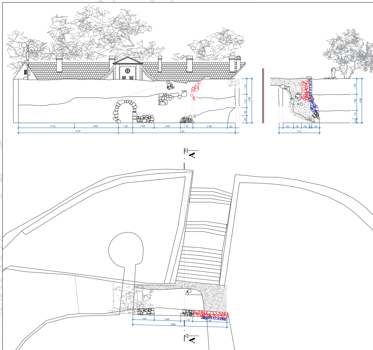
Obr. 13 Zameranie nových situácií
