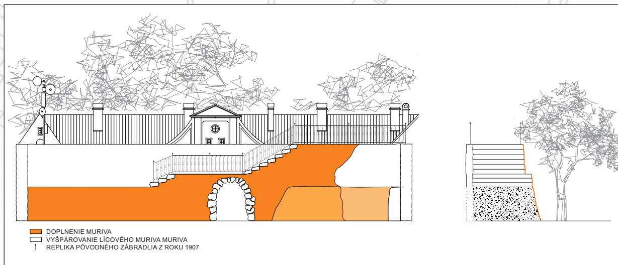
Obr. 8 Pohľad na novoveké parkové úpravy - obnova murív a schodiska
