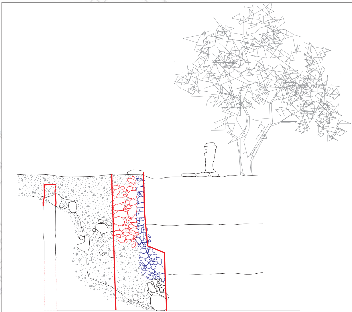
Obr. 15 Detail z realizačnej dokumentácie - schéma náhrady pôvodného staticky narušeného muriva novým, súvislým murivom, avšak v profile pôvodného muriva
