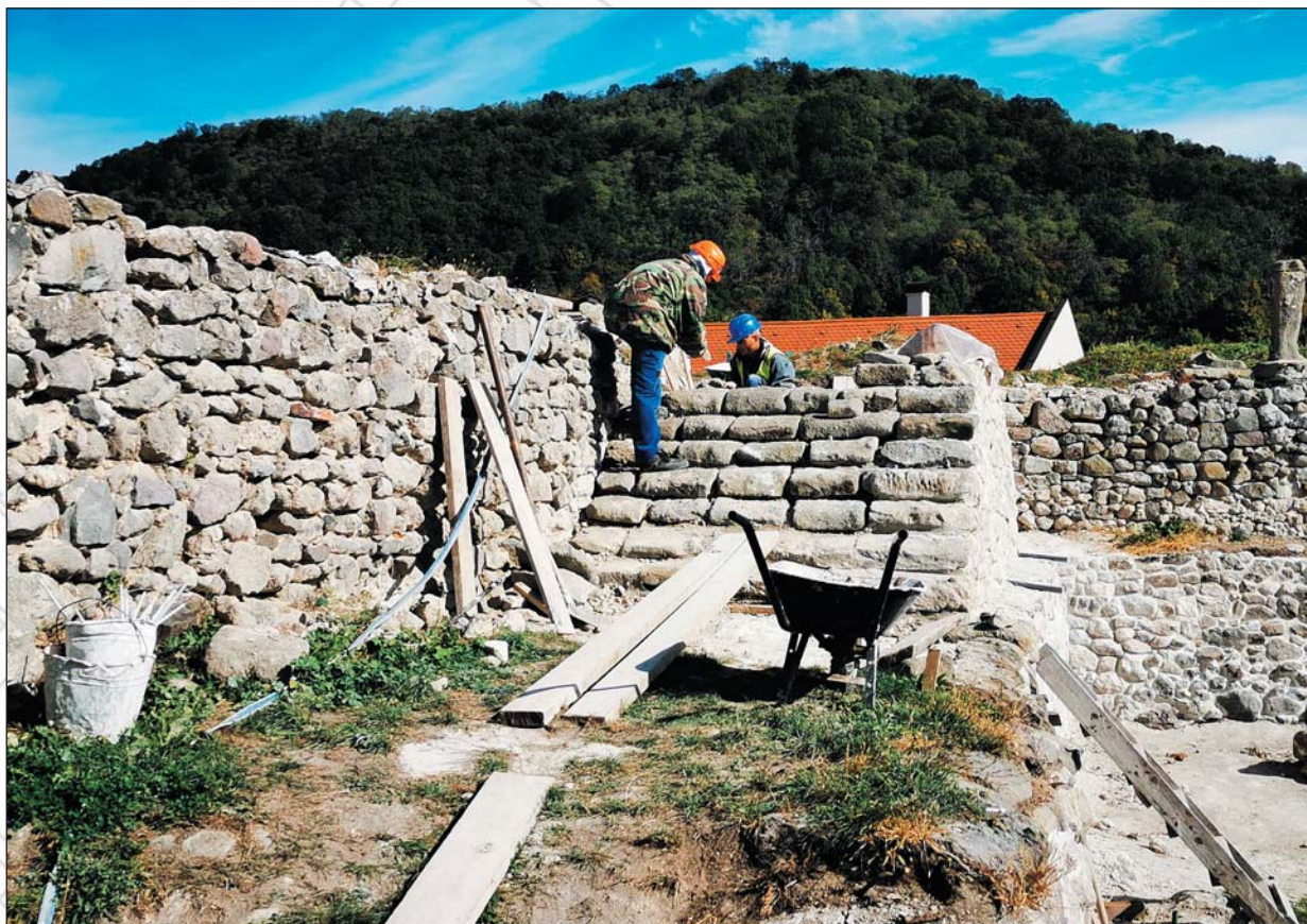
Obr. 21 Montáž schodiskových stupnic
